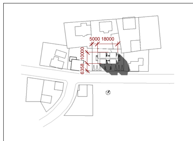
Yfirlitsmynd fyrir breytingu
