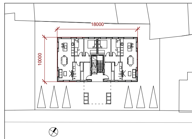
Grunnmynd 1.hæð fyrir breytingu
