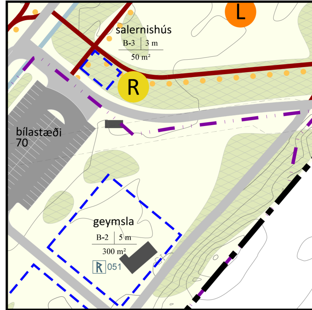
Séruppdráttur A, gildandi deiliskipulag. 1:1.000
